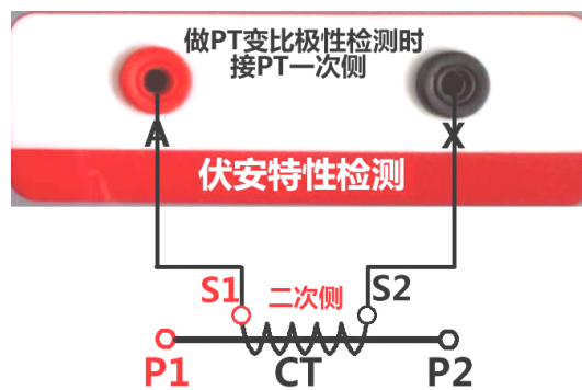
图 5 CT 励磁特性接线图
