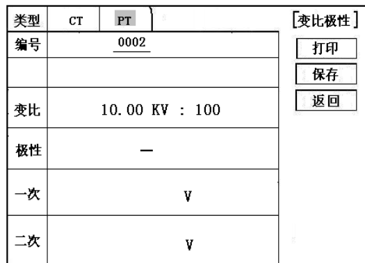
图 21 PT 变比极性测试结果界面
