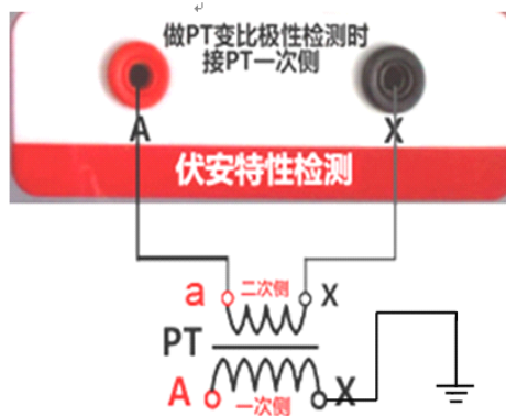
图 18 PT 励磁特性接线图
