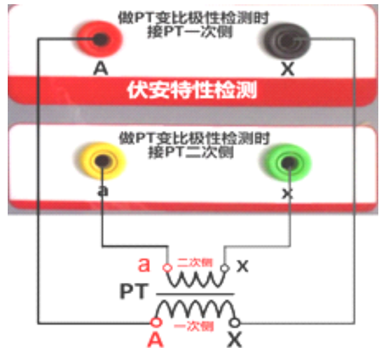
图 20 PT 变比极性接线图
