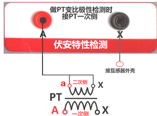
图 23 PT 交流耐压接线图
