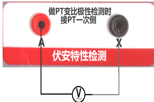
图 29, 电压校准接线图
